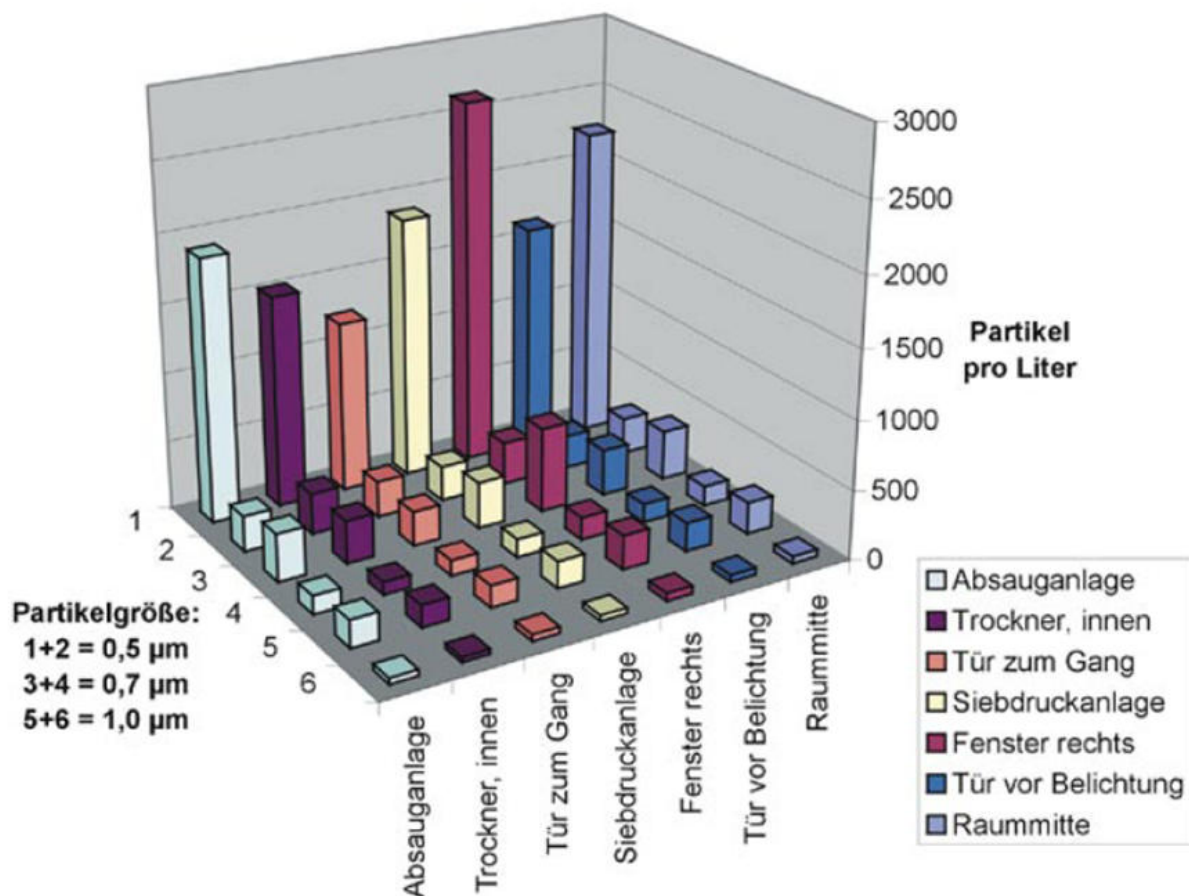
Beispiel einer Analyse vor und nach Installation eines CLAIR 2500, Luftpartikel gemessen mit METONE Partikelzähler
